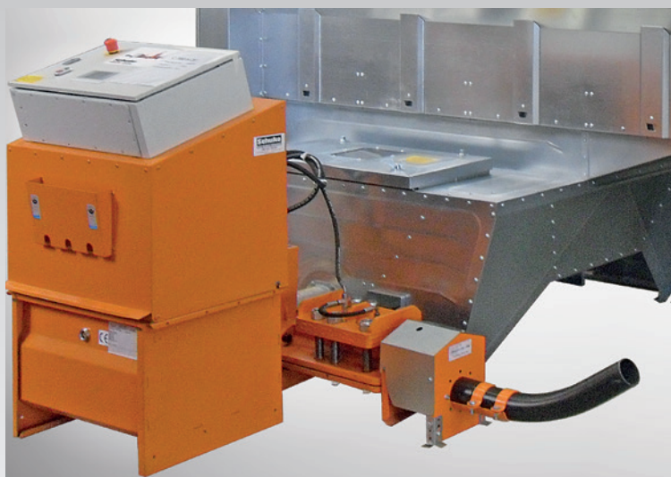
Vacomat 350 XP avec trémie SPB 100/4/130 et presse à briquettes Compacto
